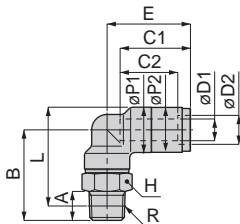
管用テーパネジの場合
